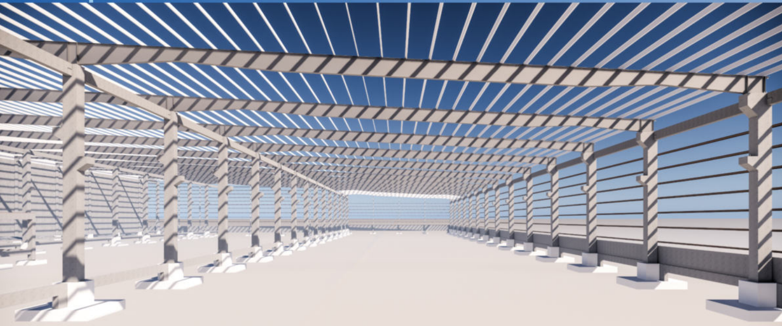
MÔ HÌNH 3D THIẾT KẾ CỘT BÊ TÔNG LẮP GHÉP, HỆ KẾT CẤU THÉP
