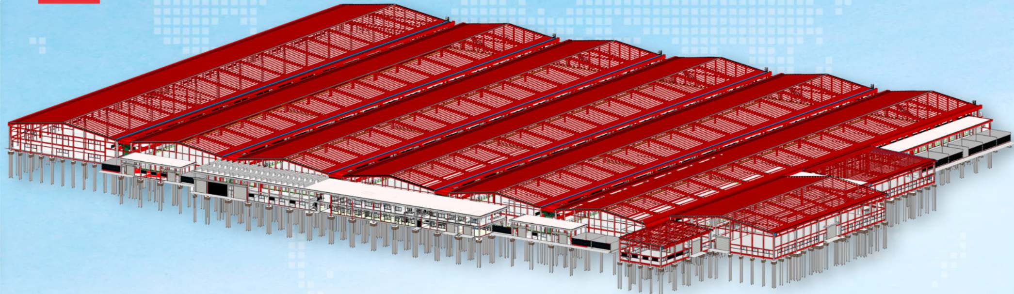
MÔ HÌNH KẾT CẤU
