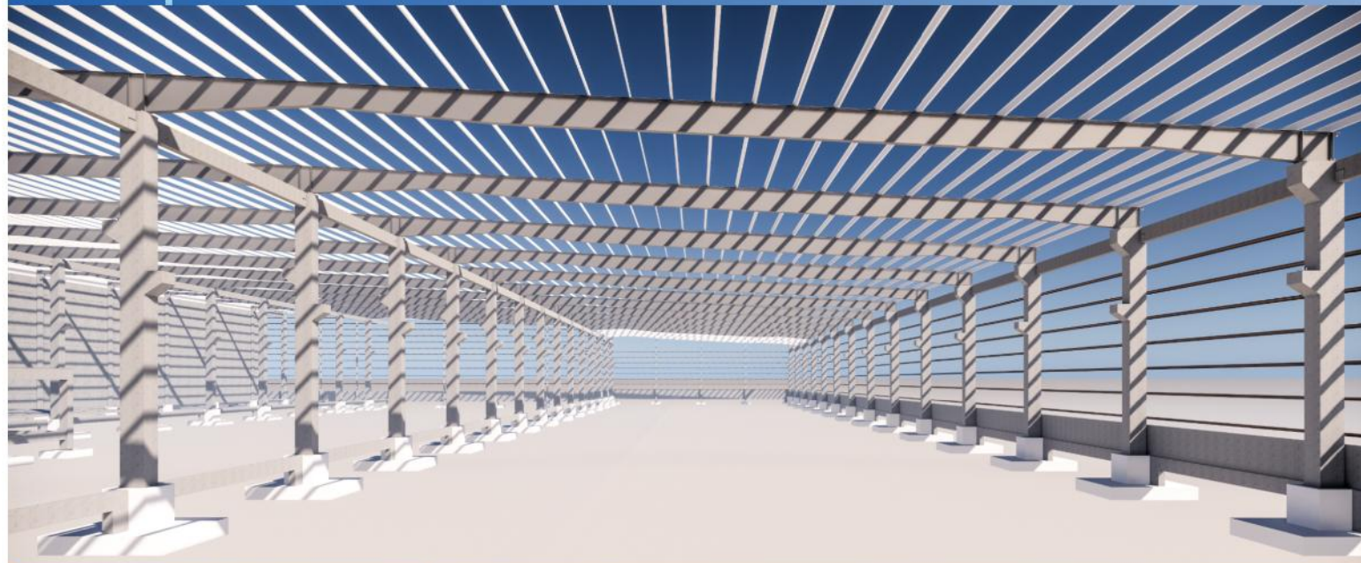
MÔ HÌNH 3D THIẾT KẾ CỘT BÊ TÔNG LẮP GHÉP, HỆ KẾT CẤU THÉP
