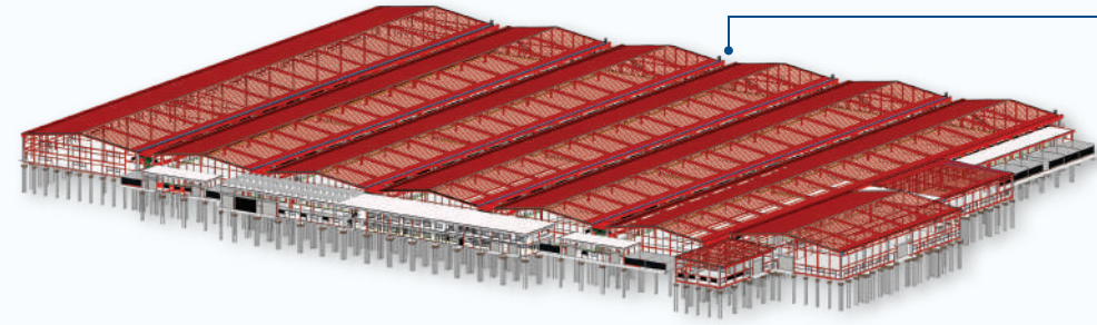
Mô hình kết cấu
